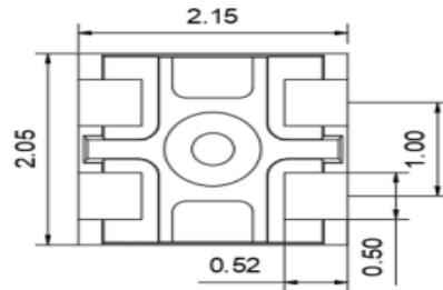
背视图 Back view
