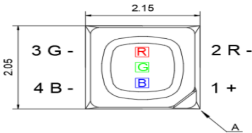
主视图 Main view
